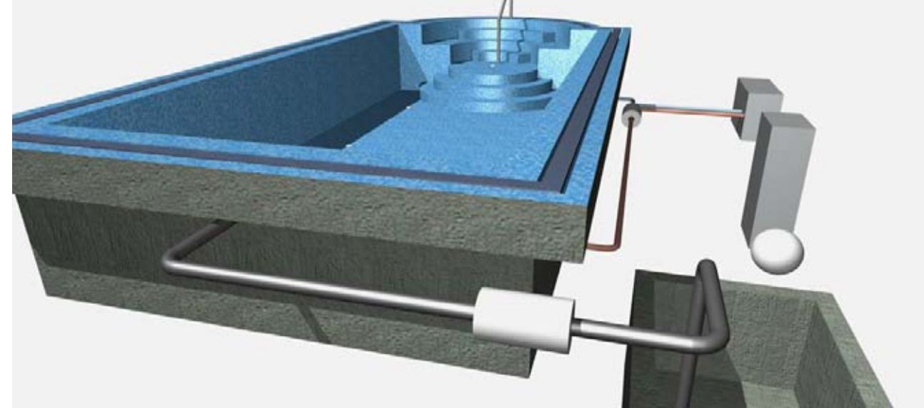
Piscina de reboso con tanque de compensación y círculo de calefacción con bomba propia
